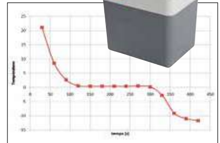
↑ Courbe de congélation de l'eau déminéralisée obtenue avec le FreezCube
